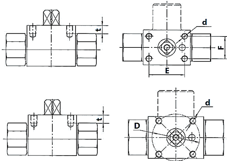
板式安装螺纹孔 (PM)
