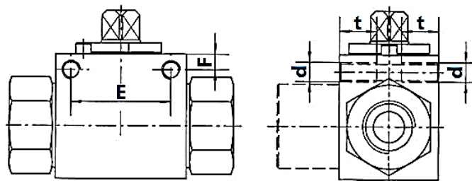
侧面双边螺纹安装孔 (TS)
